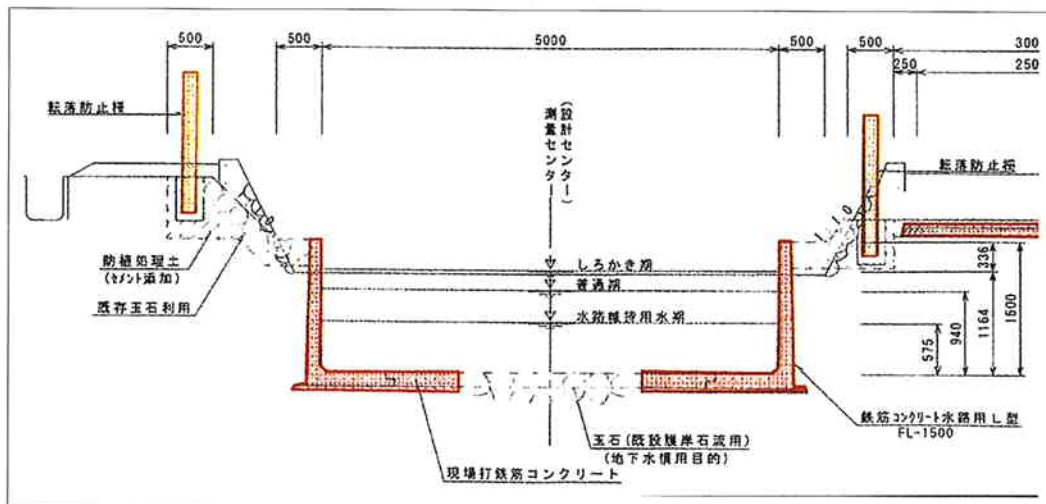
計画図
